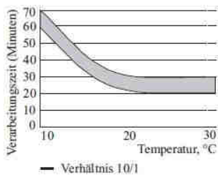
Abbildung 4: Dow Corning® 993 Dichtungsmasse – Verarbeitungszeit
