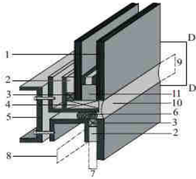
Abbildung 2: Schnitt DD: vierseitige Konstruktion - gestütztes Isolierglas
