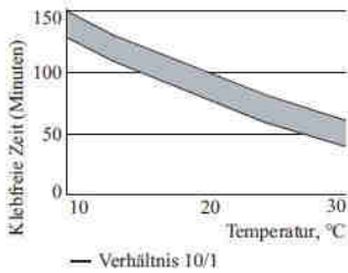
Abbildung 3: Dow Corning® 993 Dichtungsmasse – Hautbildungszeit
