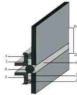
Abbildung 1B: Schnitt DD: vierseitige Konstruktion - ungestütztes Glas
