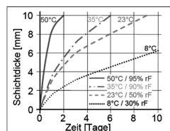
Diagramm 1: Durchhärtageschwindigkeit von 1-Komponenten Sikasil®
